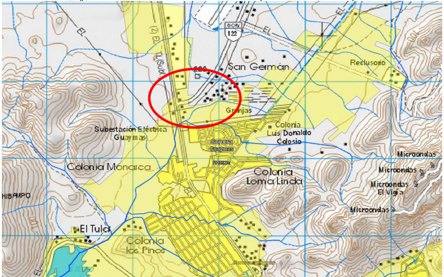
Figura 107. Punto de conflicto en el escurrimiento de arroyos en la zona norte de Guaymas
