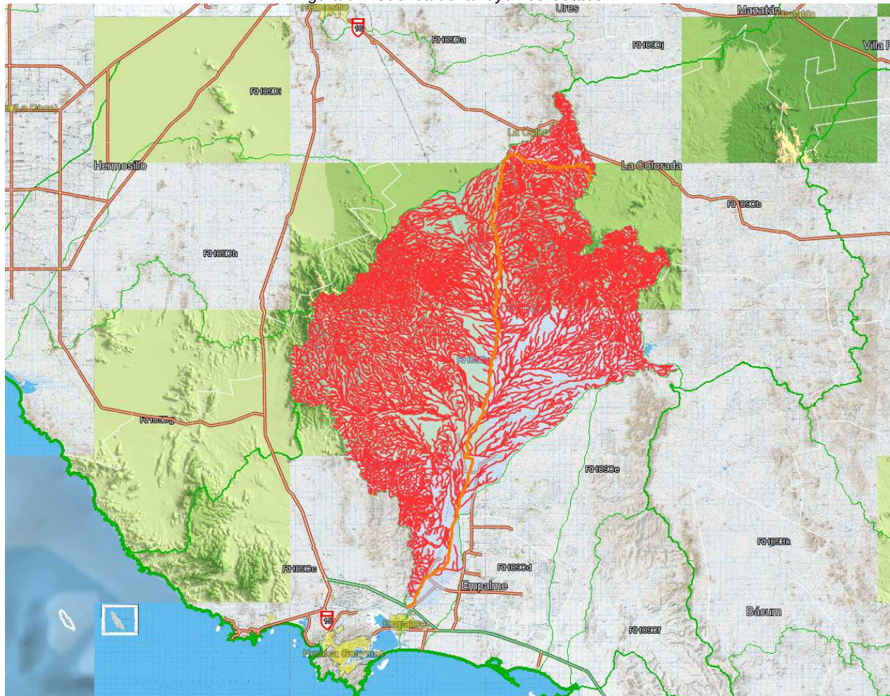
Figura 94. Cuenca del arroyo Los Cuates
