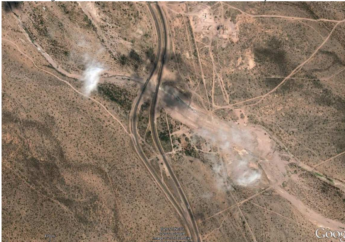
Figura 102. Puente de la carretera federal México 15 sobre el arroyo San José
