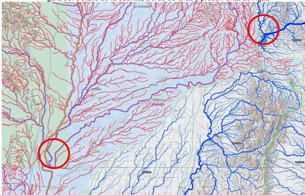
Figura 95. Detalle de la cuenca, Bordo de Ortiz y presa Punta de Agua
