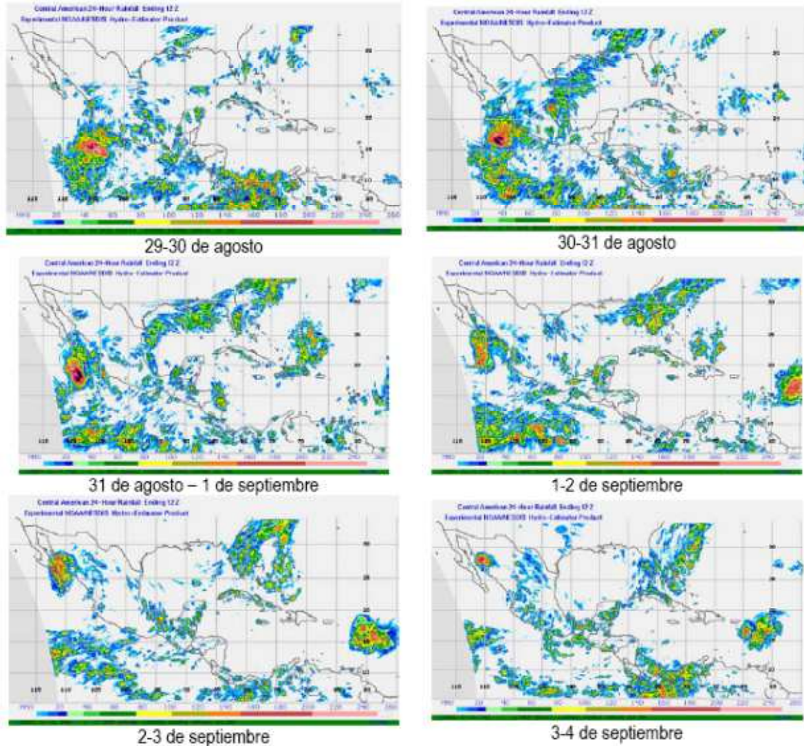
Figura 75. Secuencia diaria de “Jimena” empleando el hidroestimador de la NOAA
