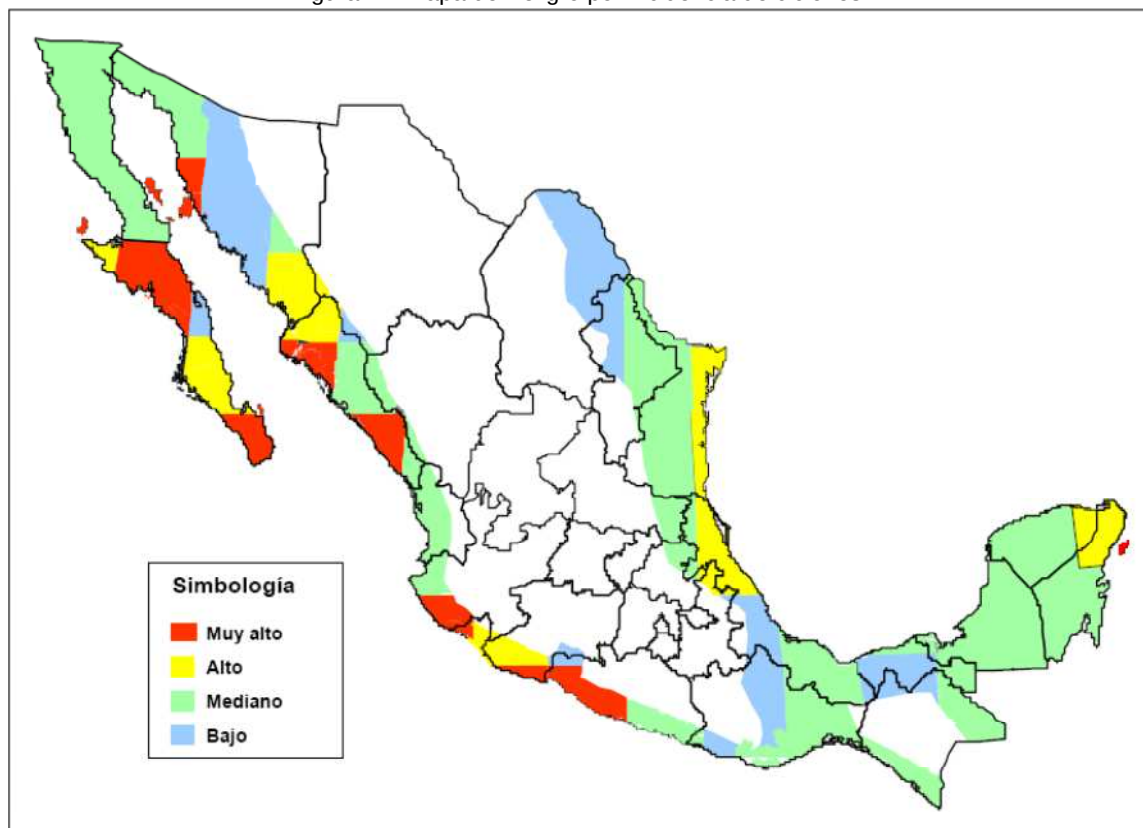
Figura 72. Mapa de Peligro por incidencia de ciclones.
