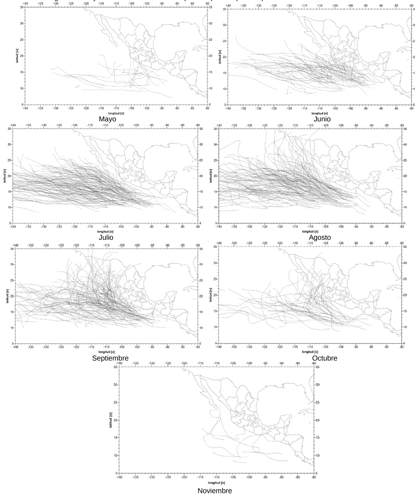
Figura 73. Trayectorias de los Ciclones Tropicales que han pasado por el Océano Pacífico de 1951 -2000
