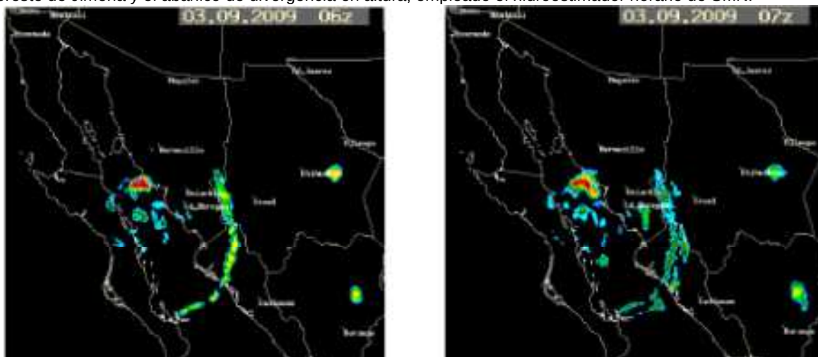
Figura 76. Secuencia Horaria del núcleo de tormenta (sobre Guaymas) asociado con la extensión del eje de vaguada localizado en el cuadrante noreste de Jimena y el abanico de divergencia en altura, empleado el hidroestimador horario de SMN.
