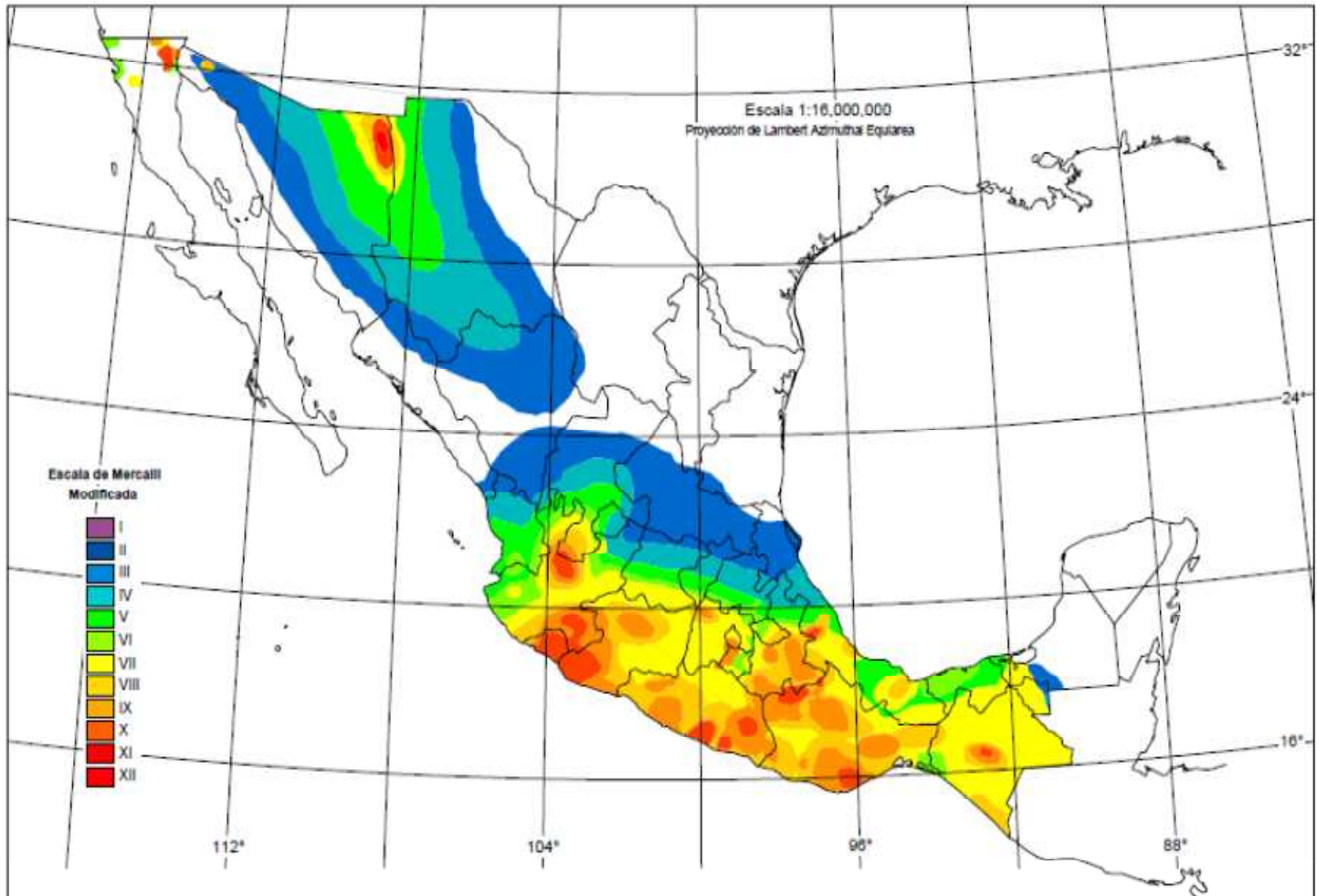
Figura 31. Mapa Global de Intensidades.
