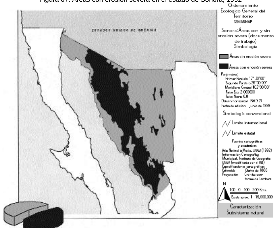
Figura 67. Áreas con erosión severa en el estado de Sonora, 1992
