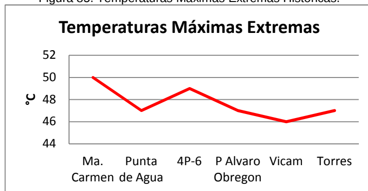
Figura 85. Temperaturas Máximas Extremas Históricas.
