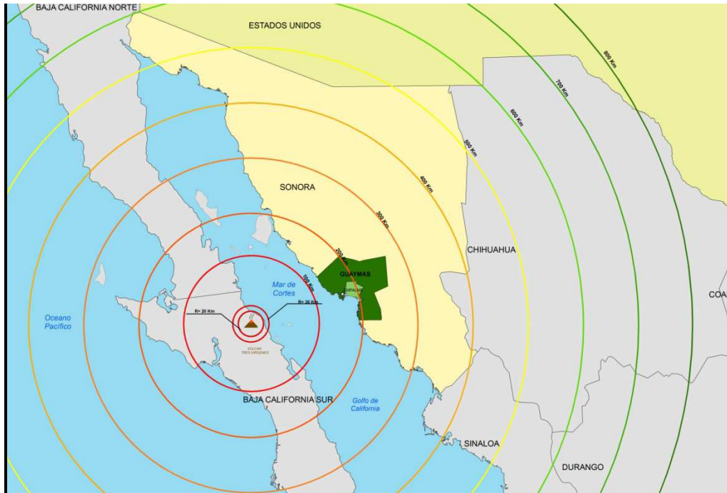
Figura 49. Ubicación regional del Volcán Tres Marías, con respecto al municipio de Guaymas.
