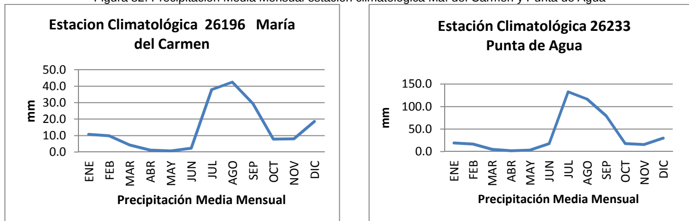
Figura 82. Precipitación Media Mensual estación climatológica Ma. del Carmen y Punta de Agua
