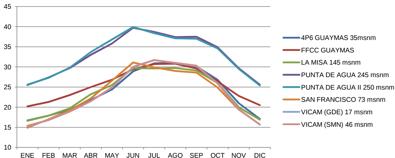
Figura 6. Temperatura Media Mensual por estación meteorológica del Municipio de Guaymas
