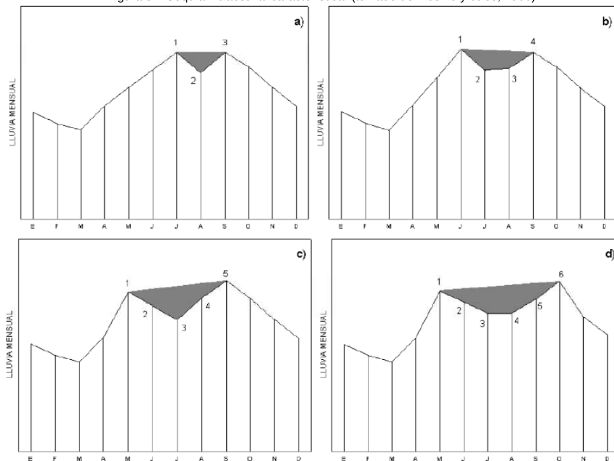
Figura 81. Sequía intraestival característica. (tomado de Mosiño y otros, 1966)
