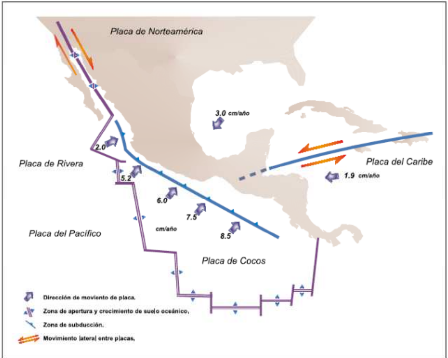
Figura 30. Placas tectónicas que afectan el territorio Mexicano.
