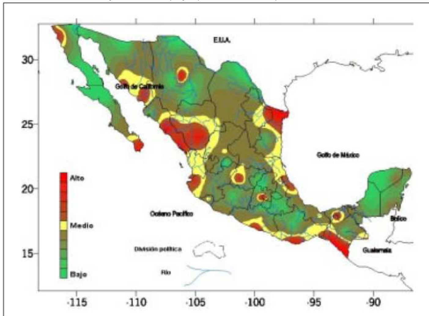
Figura 93. Zonas de peligros por inundación de la República Mexicana.
