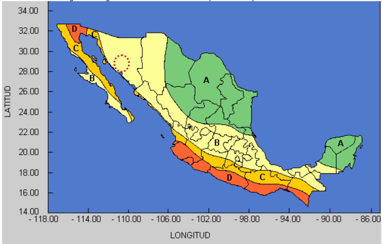
Figura 32. Regionalización Sísmica de México (Modificado a partir de Manual CFE
