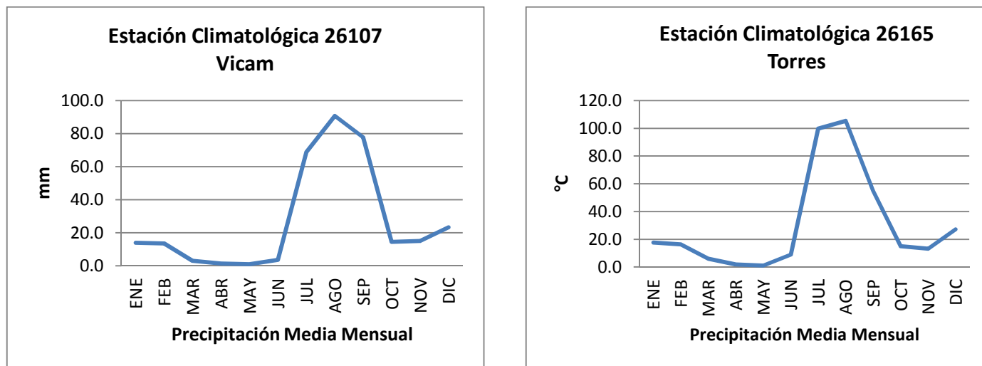
Figura 79. Precipitación Media Mensual estación climatológica Vicam y Torres
