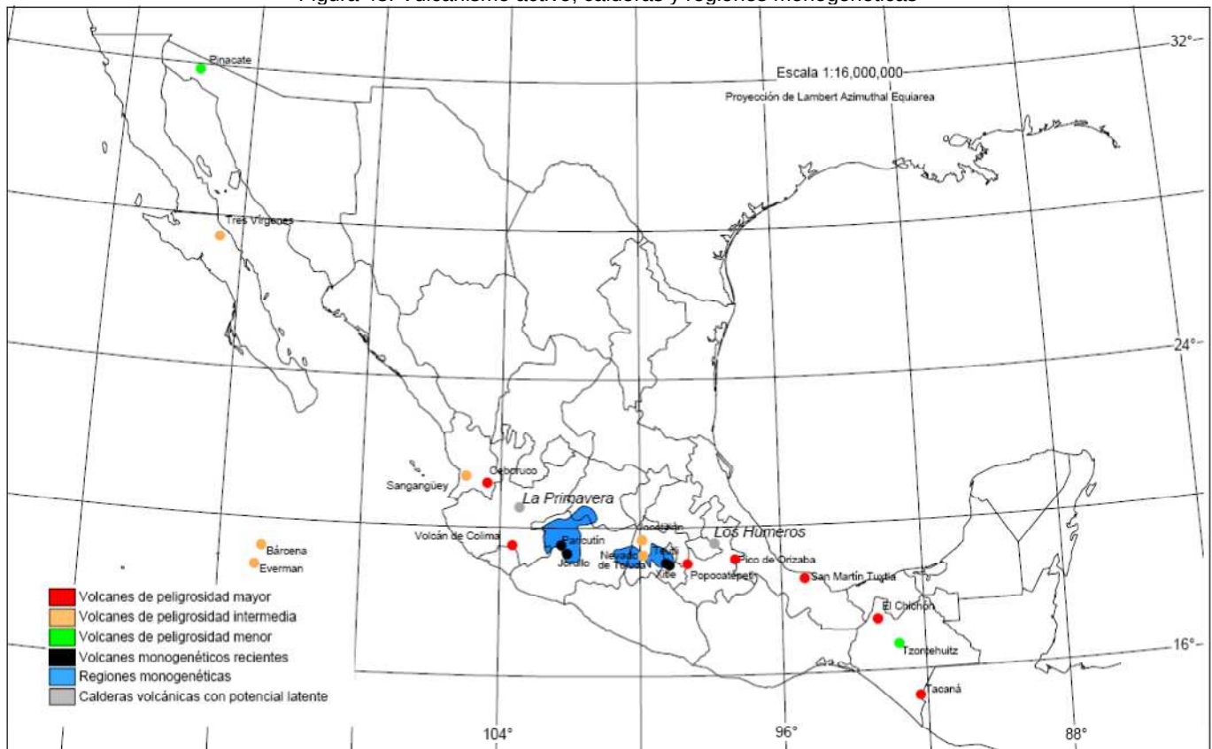
Figura 48. Vulcanismo activo, calderas y regiones monogenéticas
