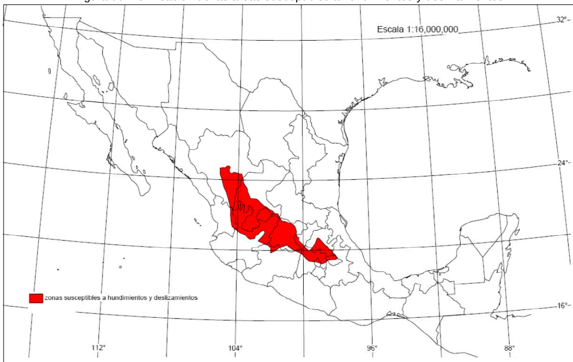
Figura 66. Zonificación de las áreas susceptibles a hundimientos y deslizamientos.
