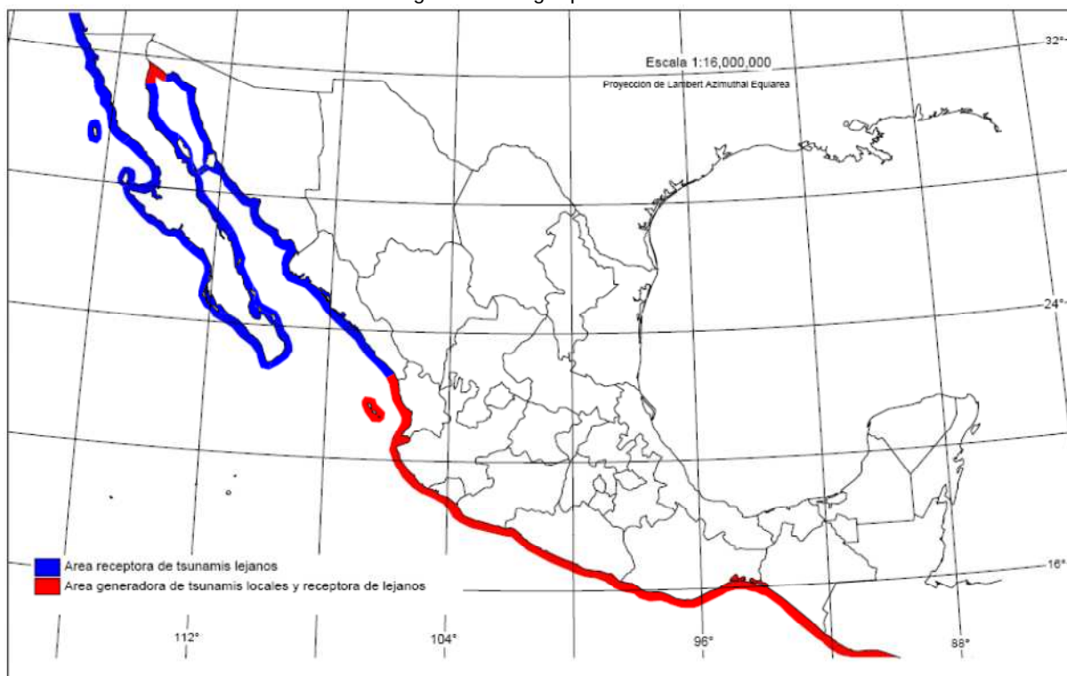
Figura 37. Peligro por Tsunami
