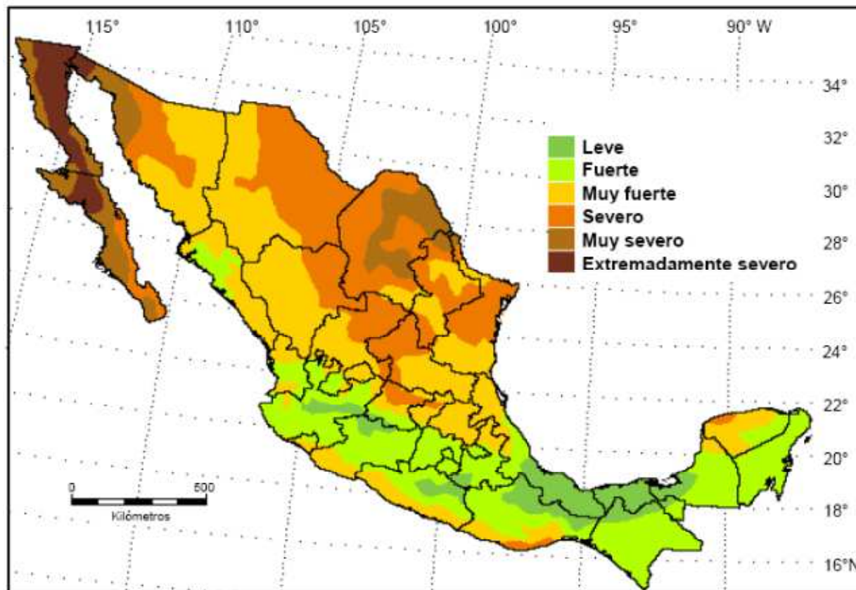
Figura 83. Índice de Severidad de la sequía meteorológica. Escenario actual.
